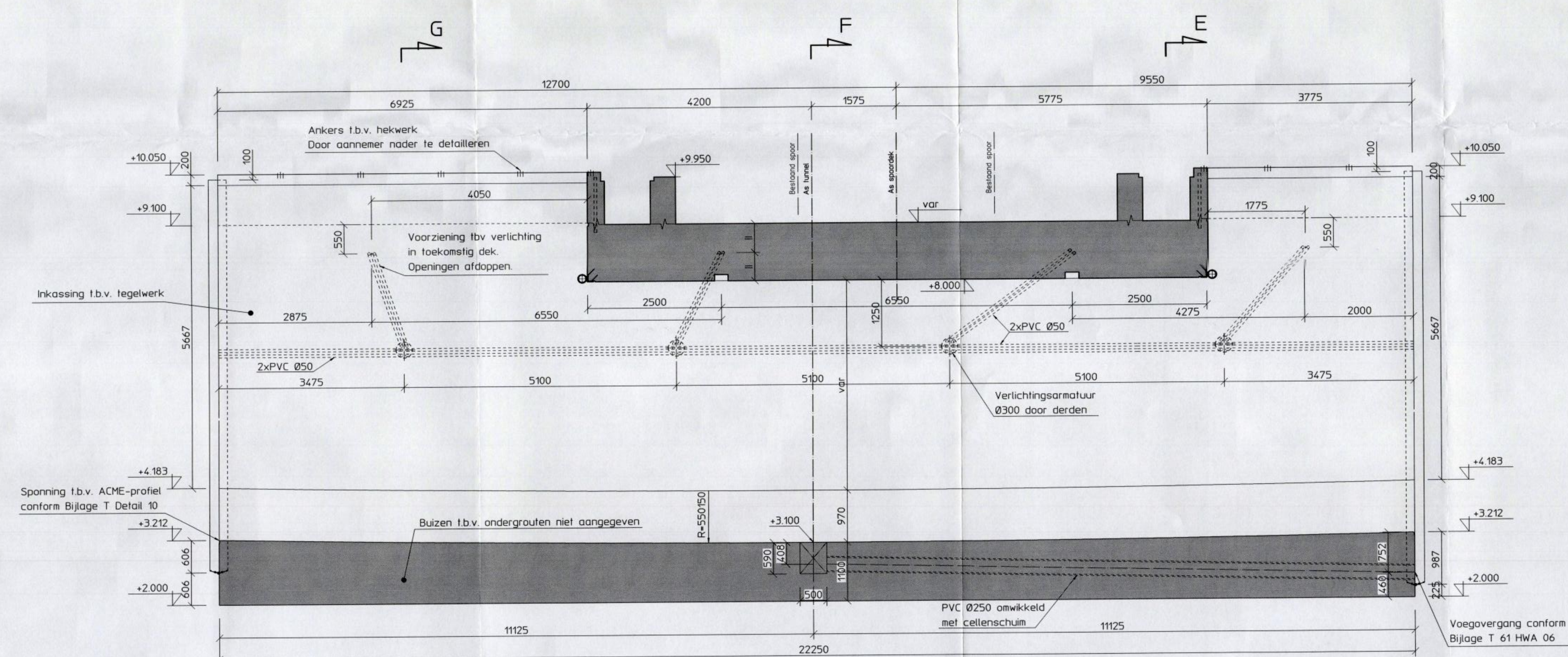
Doorsnede C
