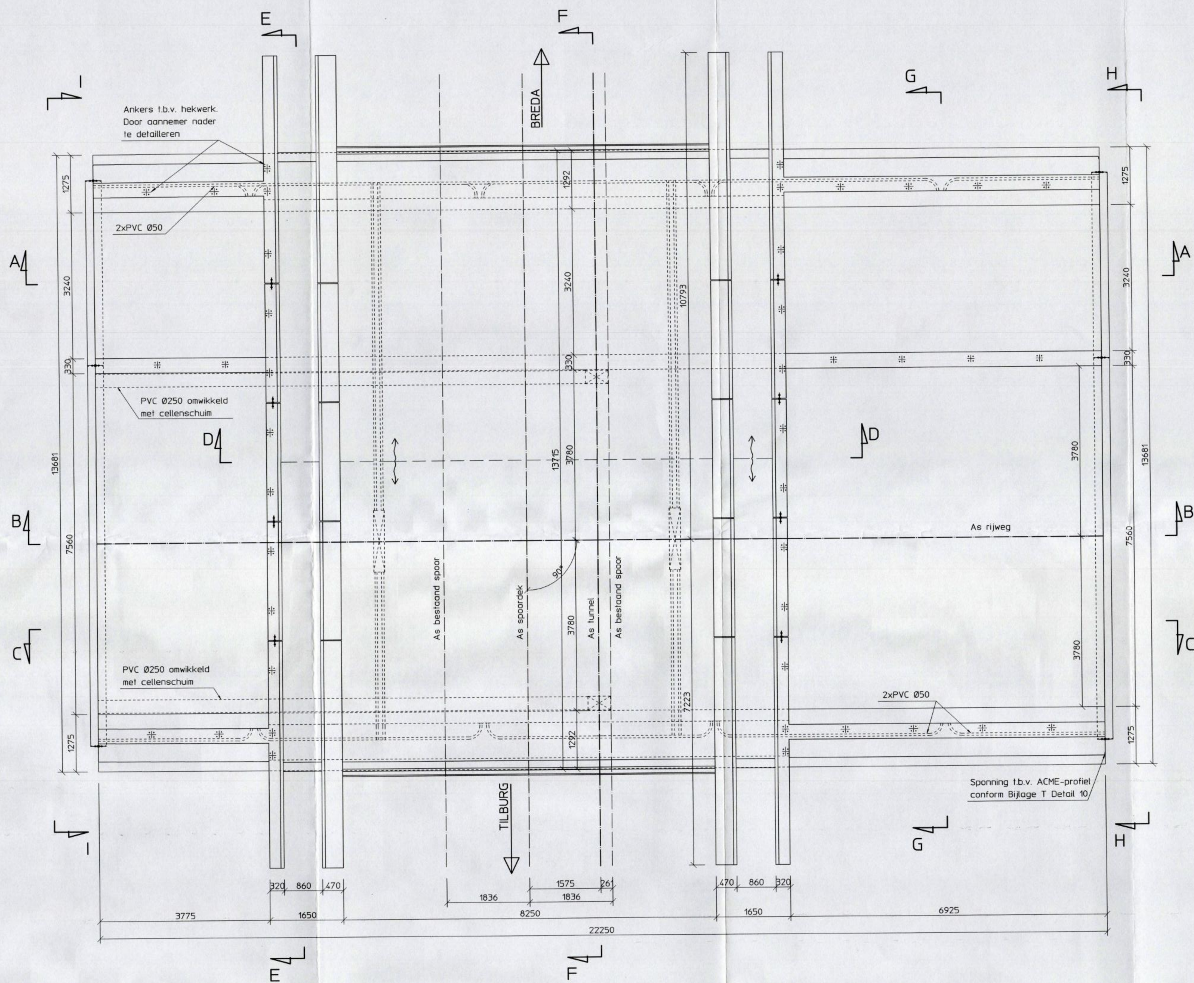
Bovenaanzicht
