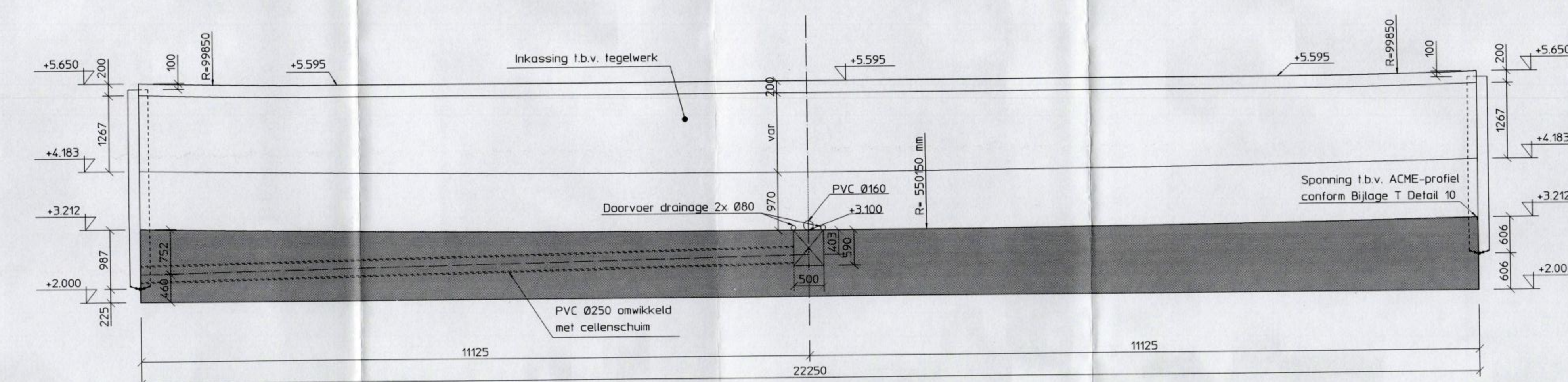
Doorsnede B
