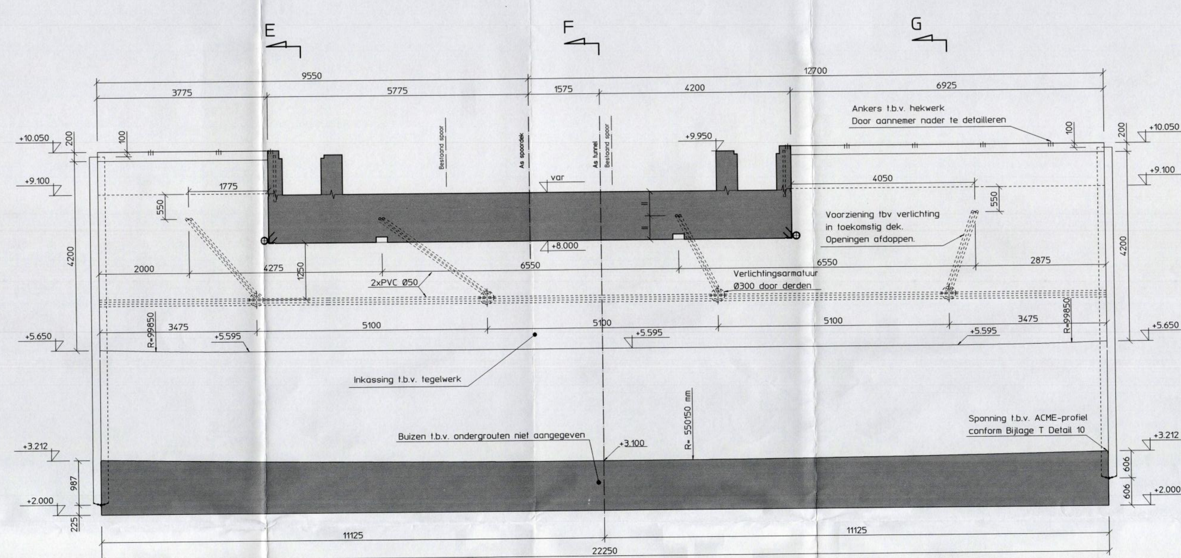
Doorsnede A
